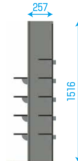
< 側面図 >
